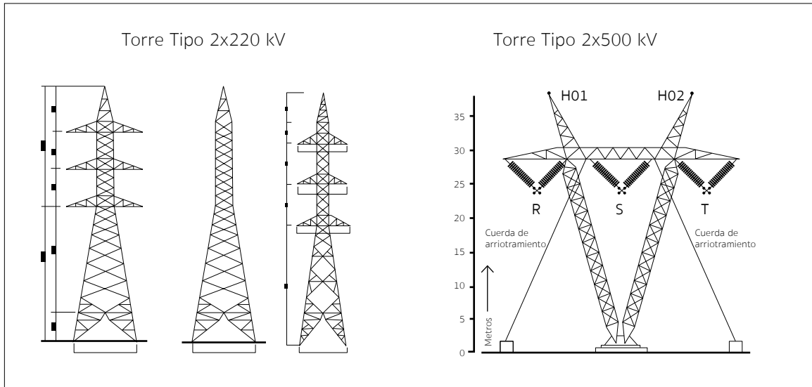
Figura 8. Siluetas de Estructuras utilizadas en LTx.
